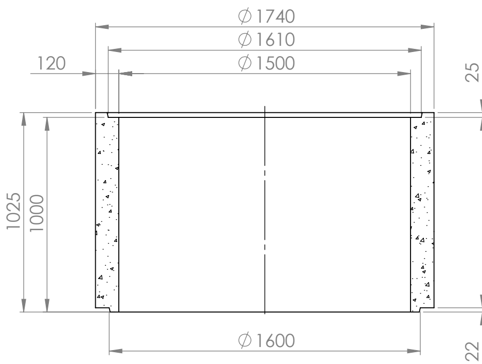
KESKILINJAN LEIKKAUS
