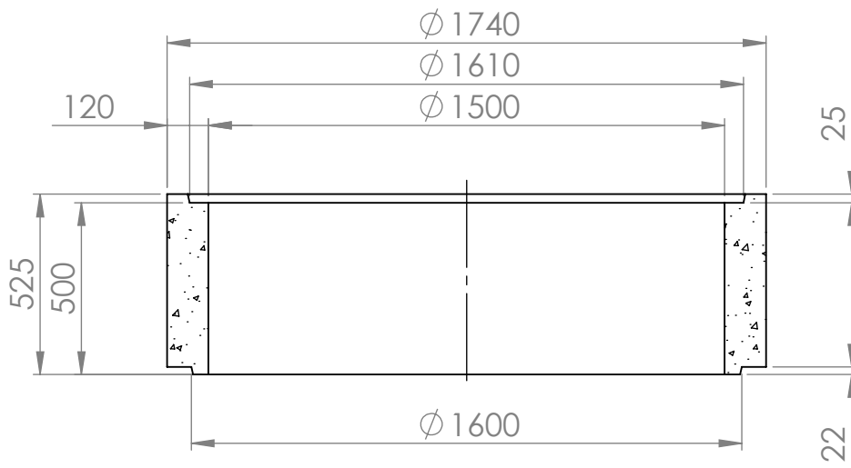
KESKILINJAN LEIKKAUS
