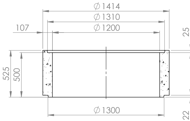
KESKILINJAN LEIKKAUS
