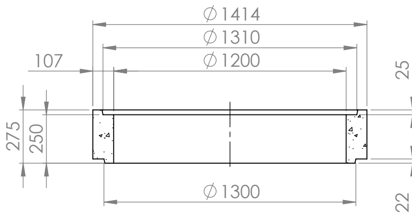
KESKILINJAN LEIKKAUS
