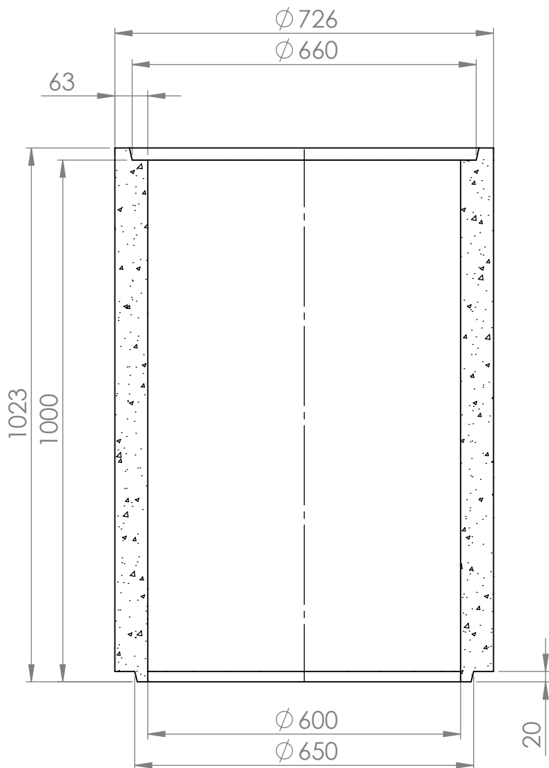
KESKILINJAN LEIKKAUS
