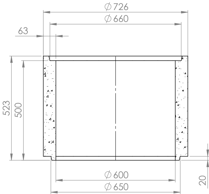
KESKILINJAN LEIKKAUS
