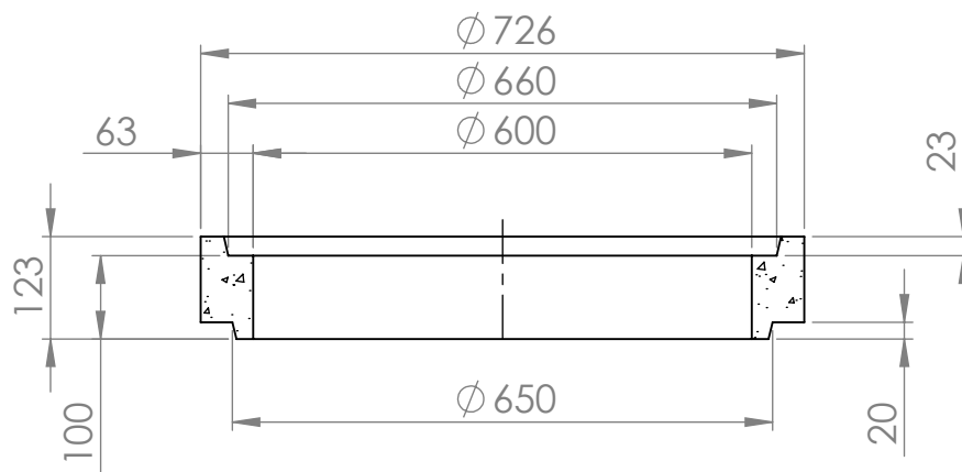
KESKILINJAN LEIKKAUS
