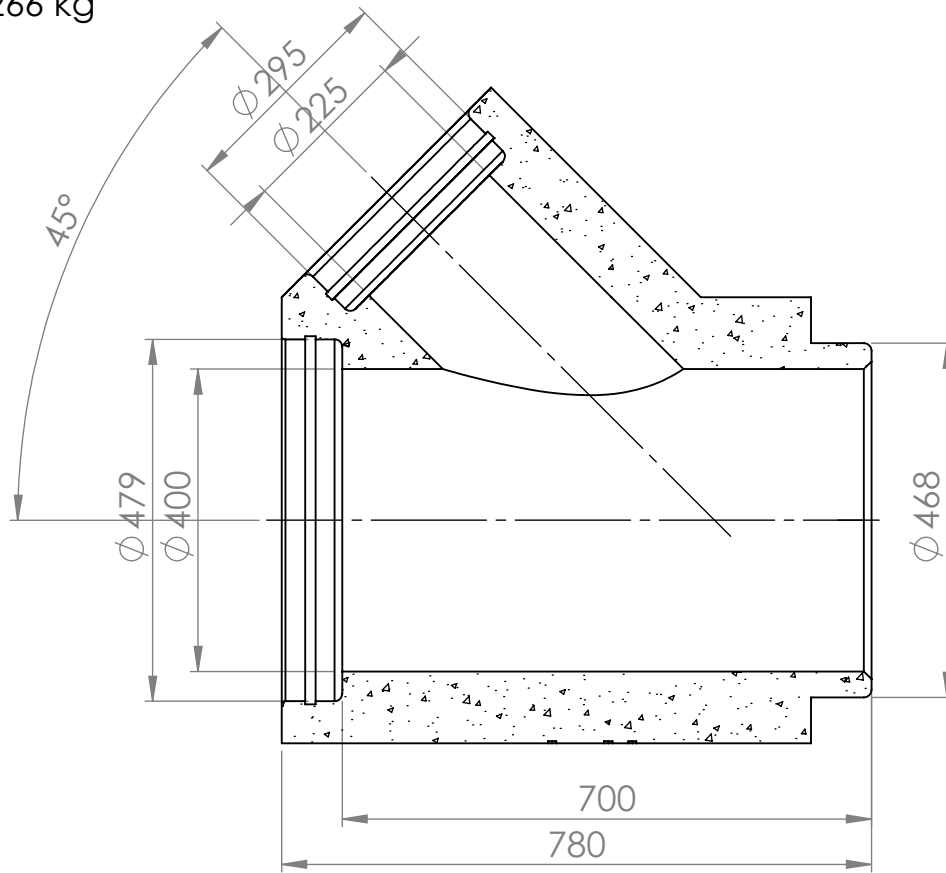
LEIKKAUS A-A
