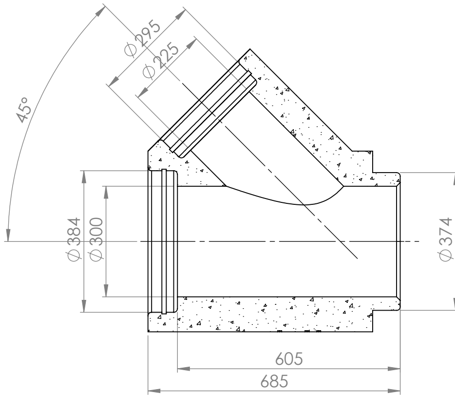
LEIKKAUS A-A
