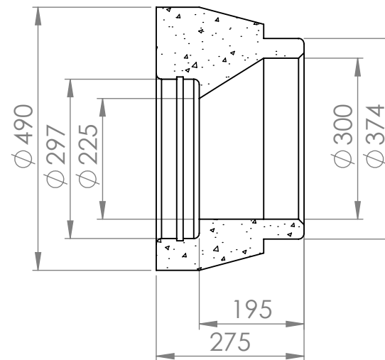
LEIKKAUS A-A
