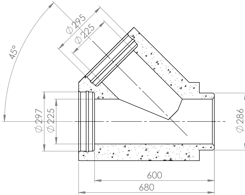
LEIKKAUS A-A
