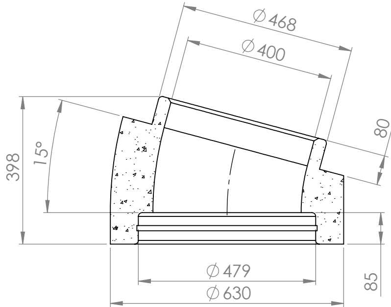
LEIKKAUS A-A
