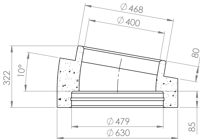
LEIKKAUS A-A
