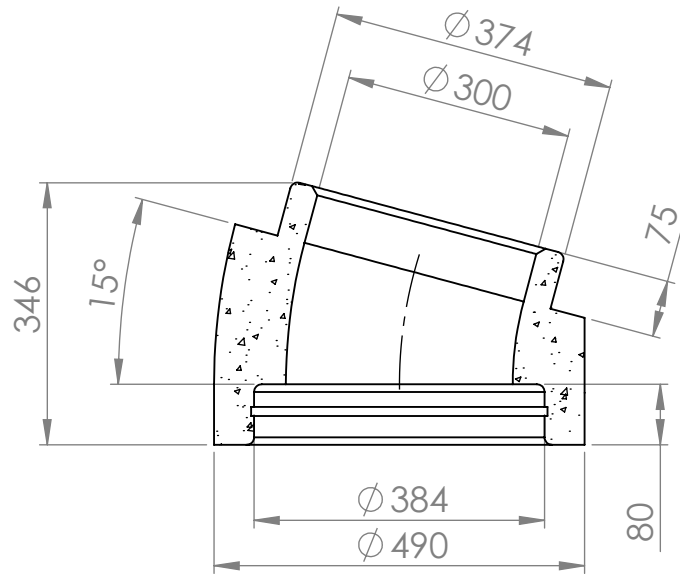
LEIKKAUS A-A
