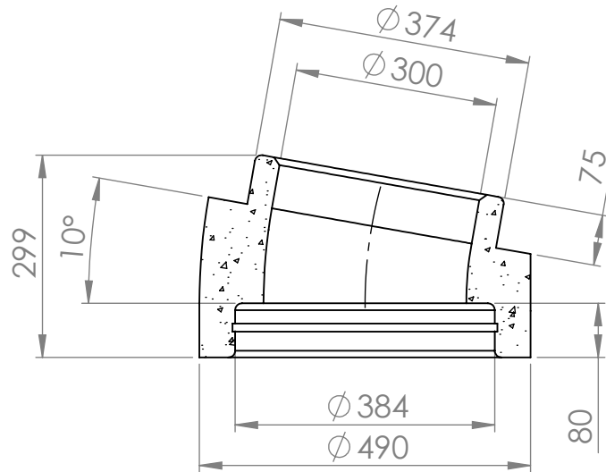
LEIKKAUS A-A
