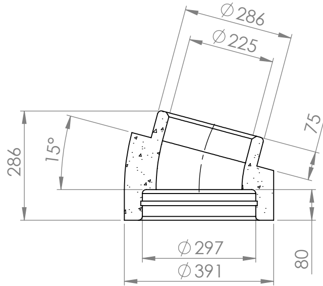
LEIKKAUS A-A
