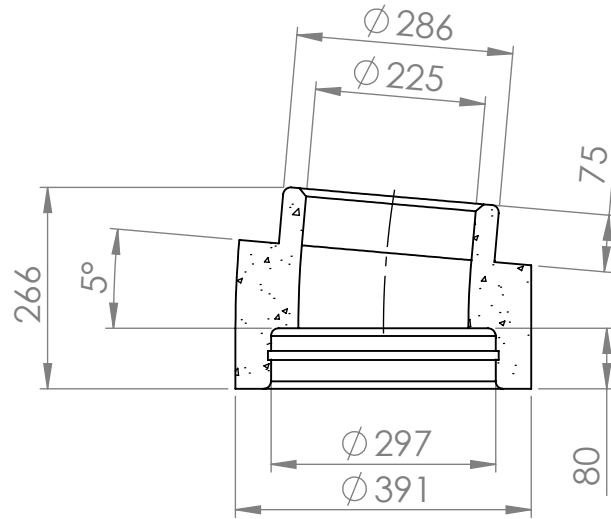
LEIKKAUS A-A
