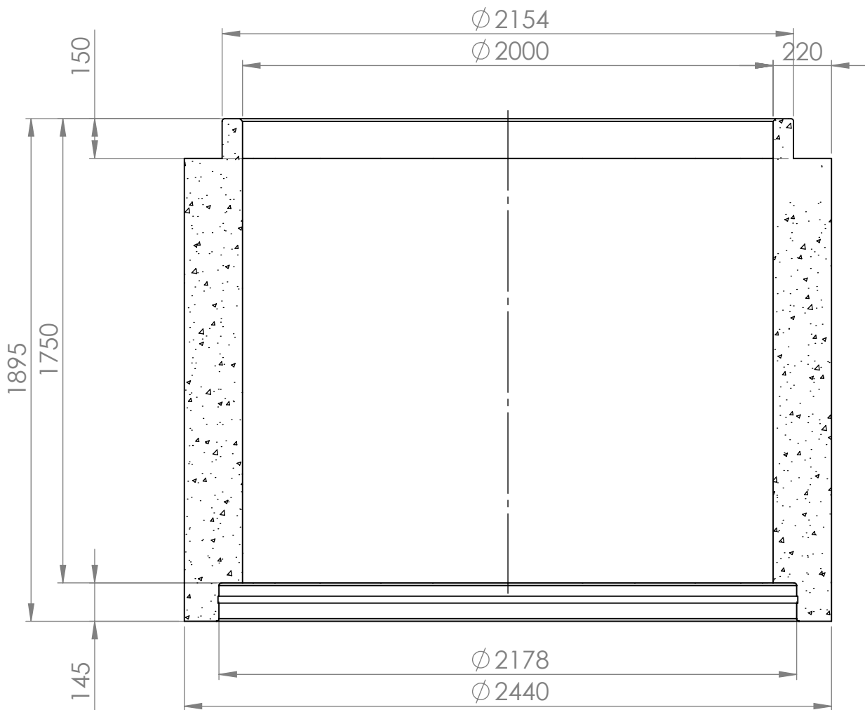
KESKILINJAN LEIKKAUS
