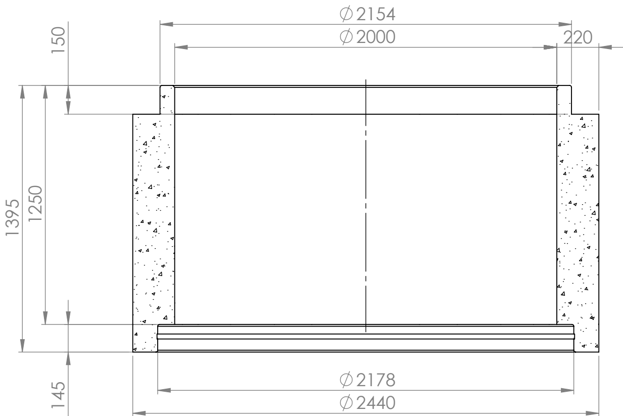
KESKILINJAN LEIKKAUS
