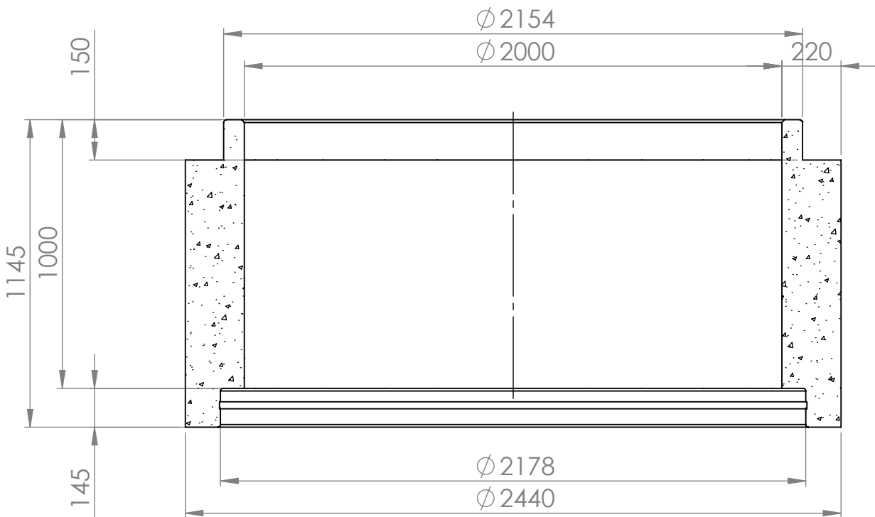
KESKILINJAN LEIKKAUS
