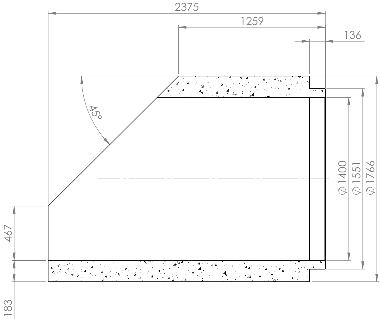
KESKILINJAN LEIKKAUS
