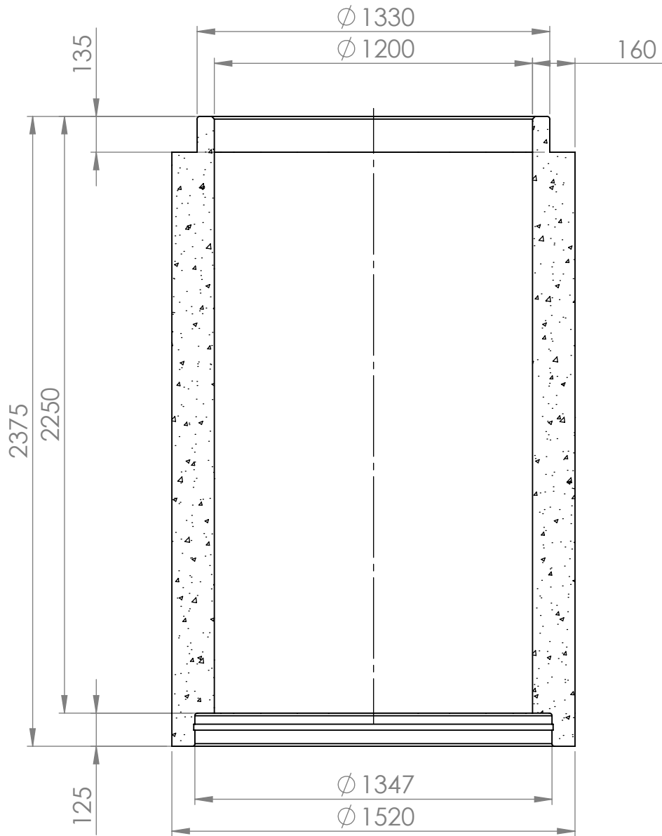
KESKILINJAN LEIKKAUS
