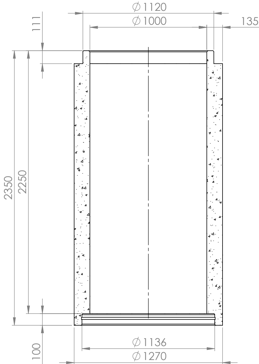
KESKILINJAN LEIKKAUS
