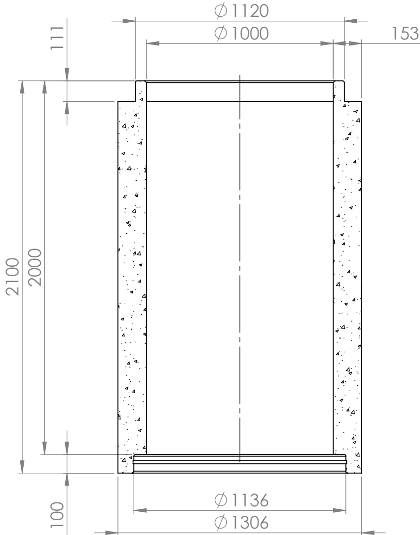
KESKILINJAN LEIKKAUS
