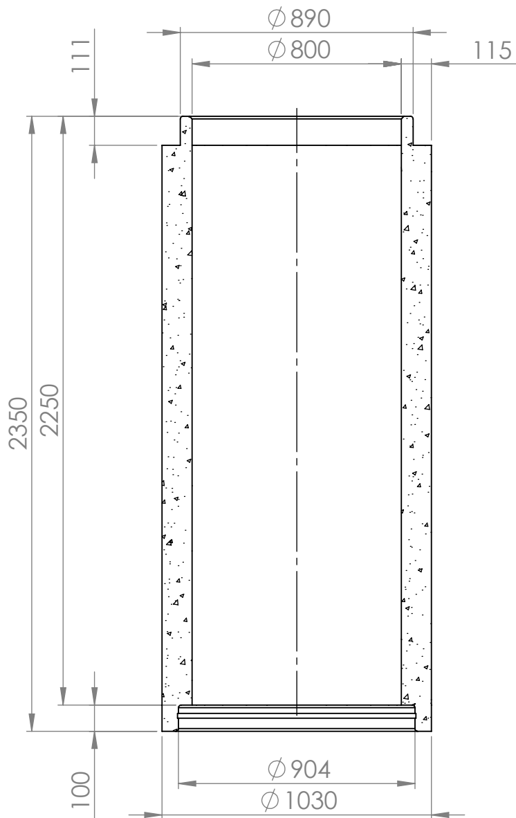
KESKILINJAN LEIKKAUS
