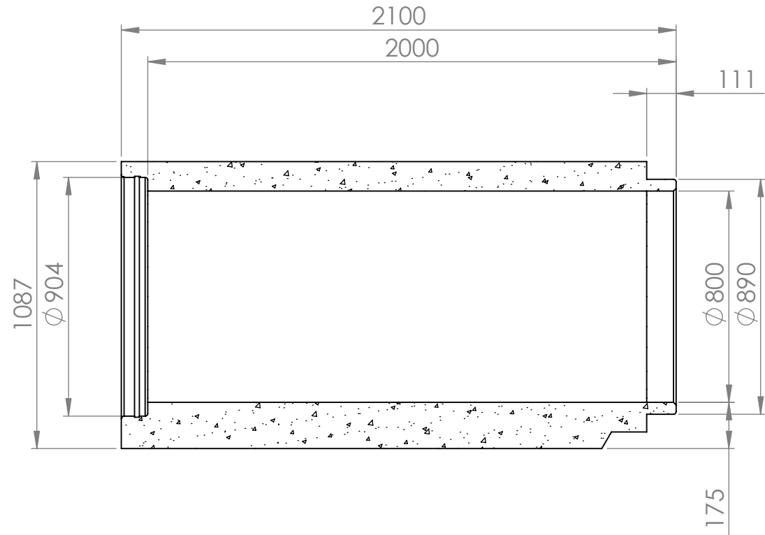
LEIKKAUS A-A
