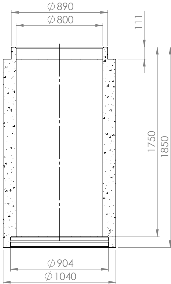
KESKILINJAN LEIKKAUS
