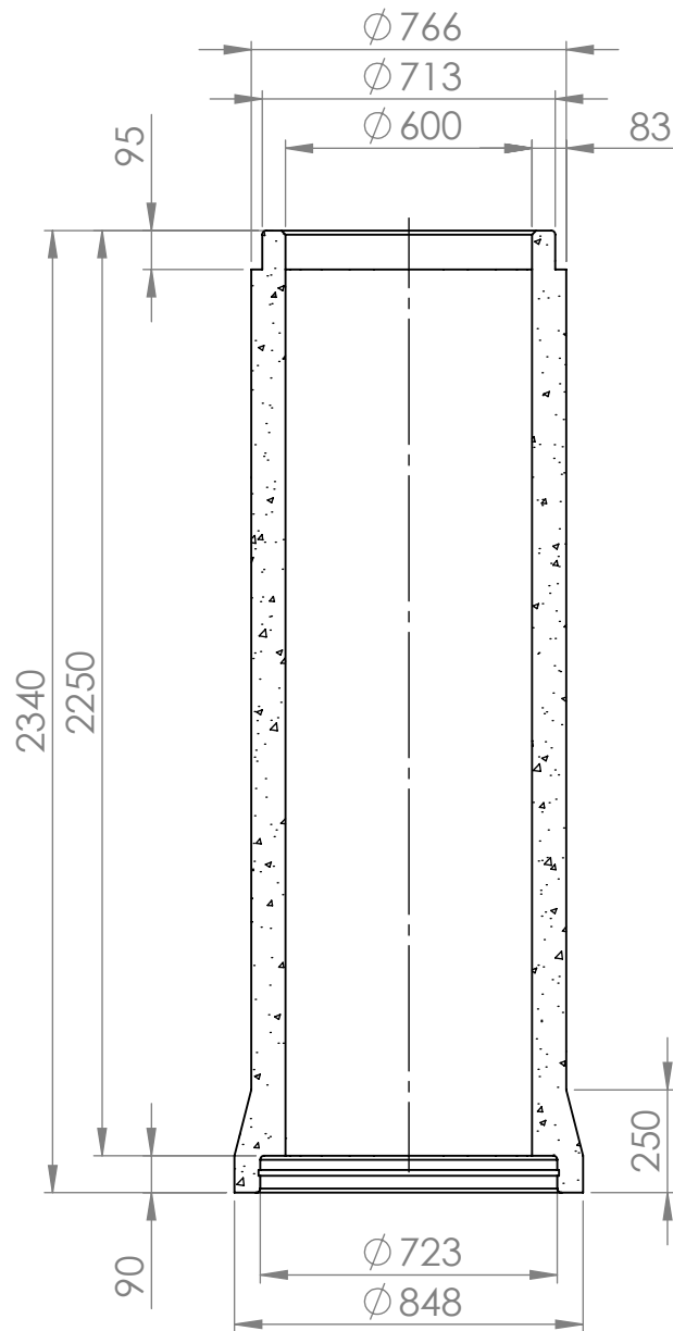
KESKILINJAN LEIKKAUS
