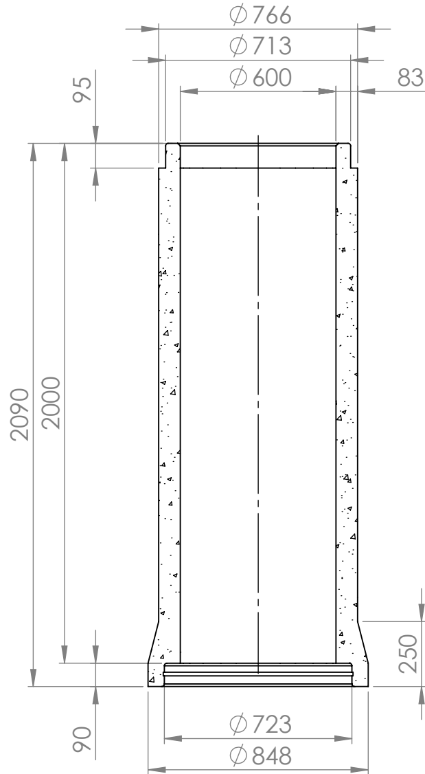
KESKILINJAN LEIKKAUS
