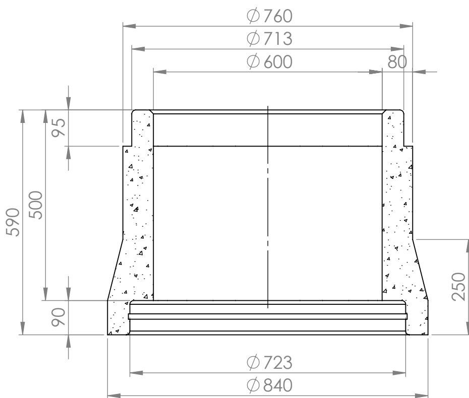
KESKILINJAN LEIKKAUS
