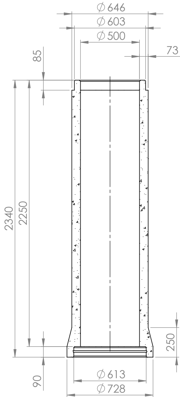
KESKILINJAN LEIKKAUS
