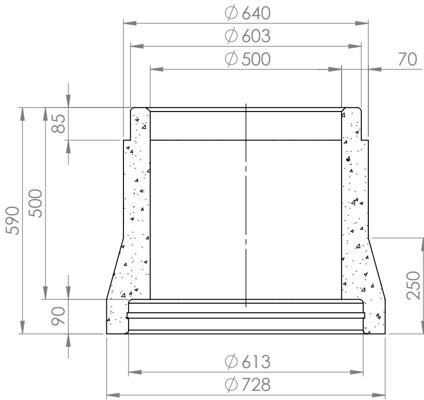
KESKILINJAN LEIKKAUS
