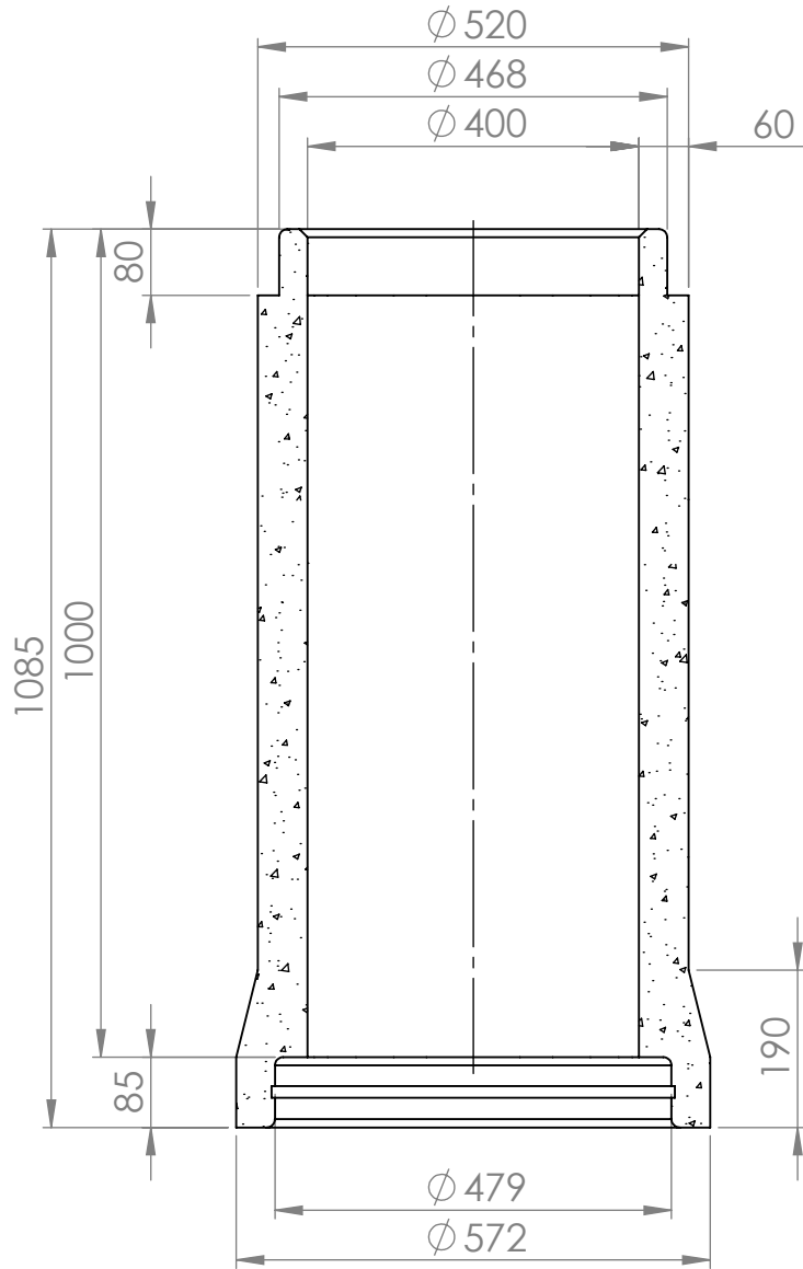
KESKILINJAN LEIKKAUS
