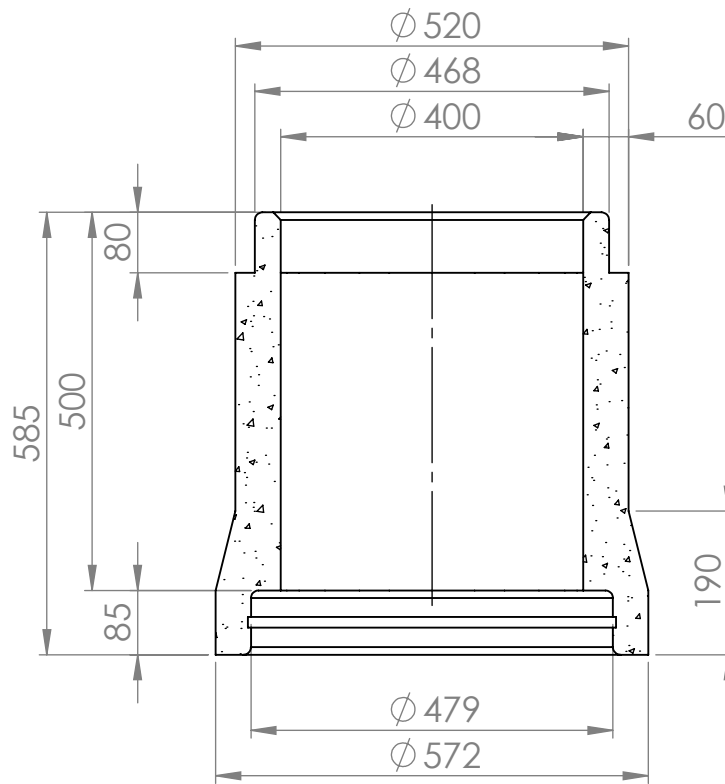
KESKILINJAN LEIKKAUS
