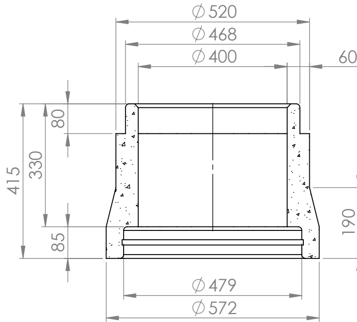
KESKILINJAN LEIKKAUS
