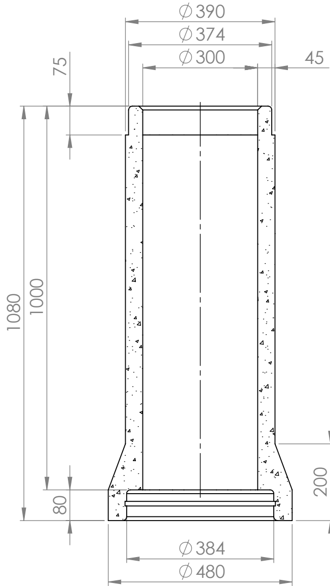
KESKILINJAN LEIKKAUS
