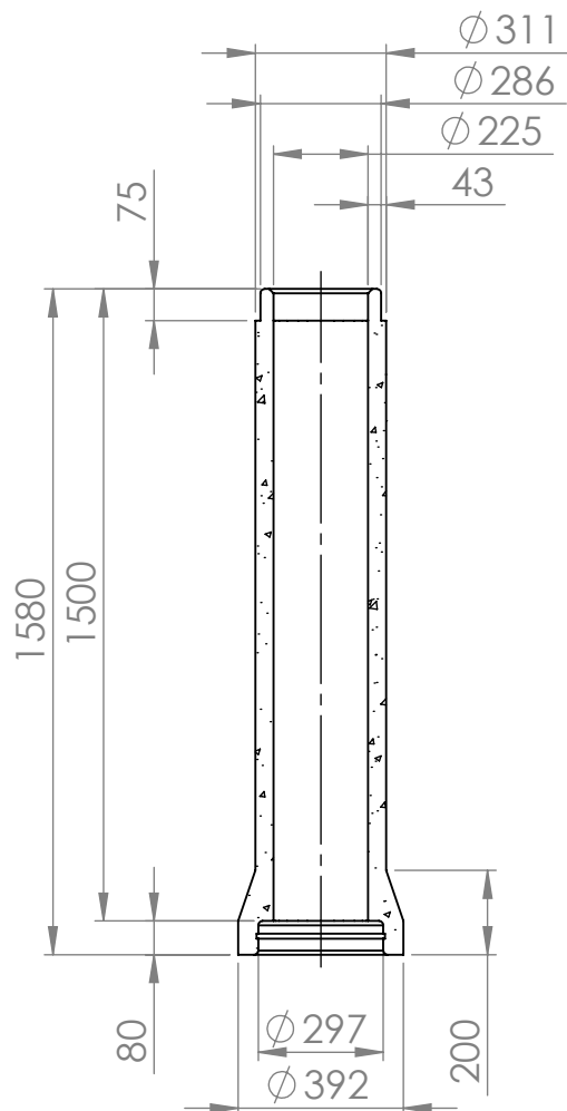
KESKILINJAN LEIKKAUS
