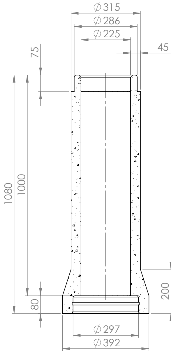
KESKILINJAN LEIKKAUS
