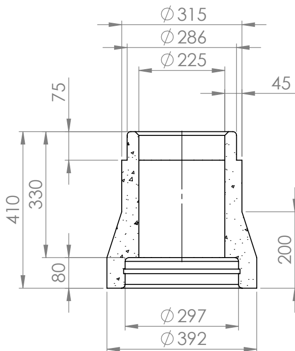
KESKILINJAN LEIKKAUS
