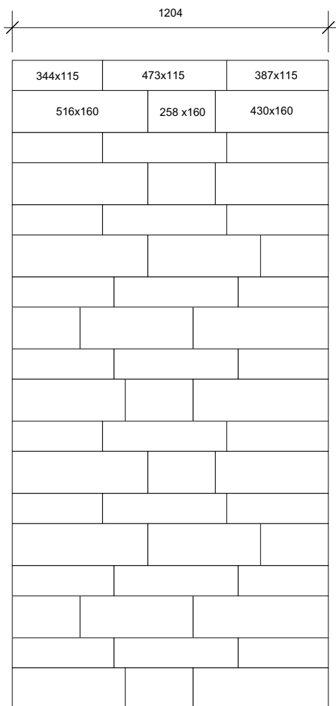
Käytäväladonta leveys 1204 mm
