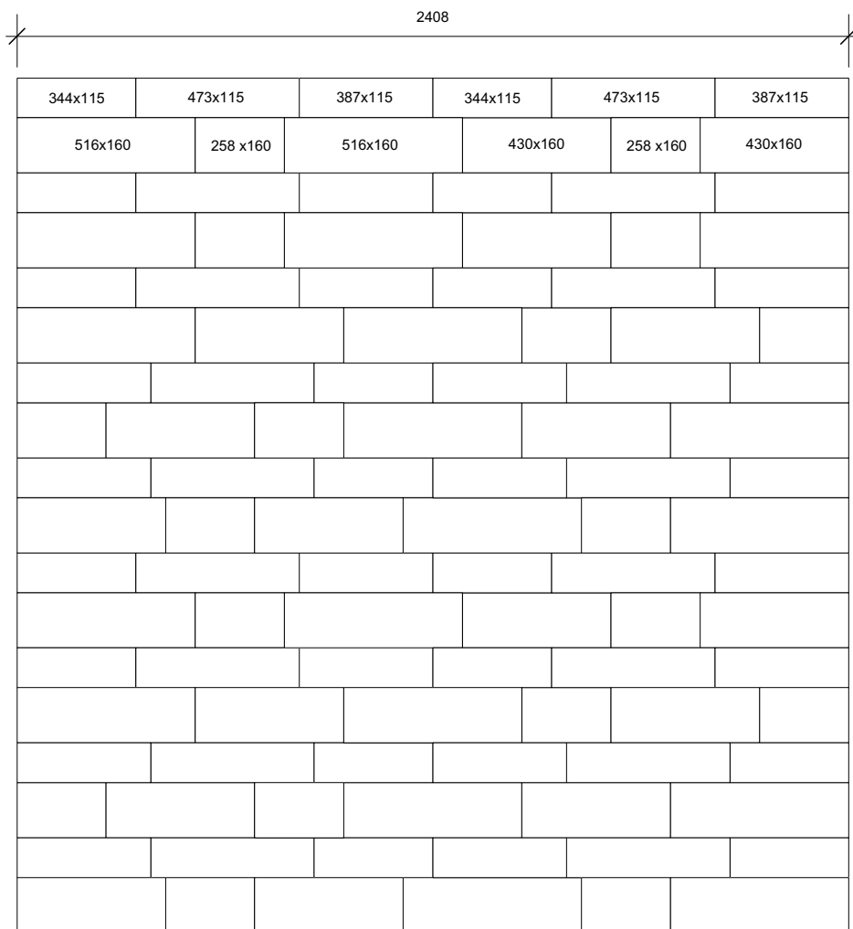
Käytäväladonta leveys 1408 mm
