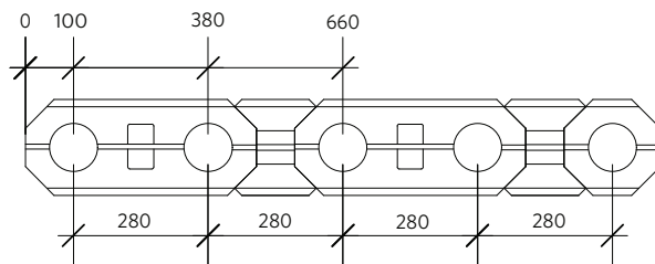
Aitakivi - raudoituksen mitoitus muurin päästä
