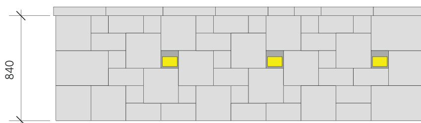
Paasikko muuri, roomalainen ladonta h=840 mm valaisimilla
